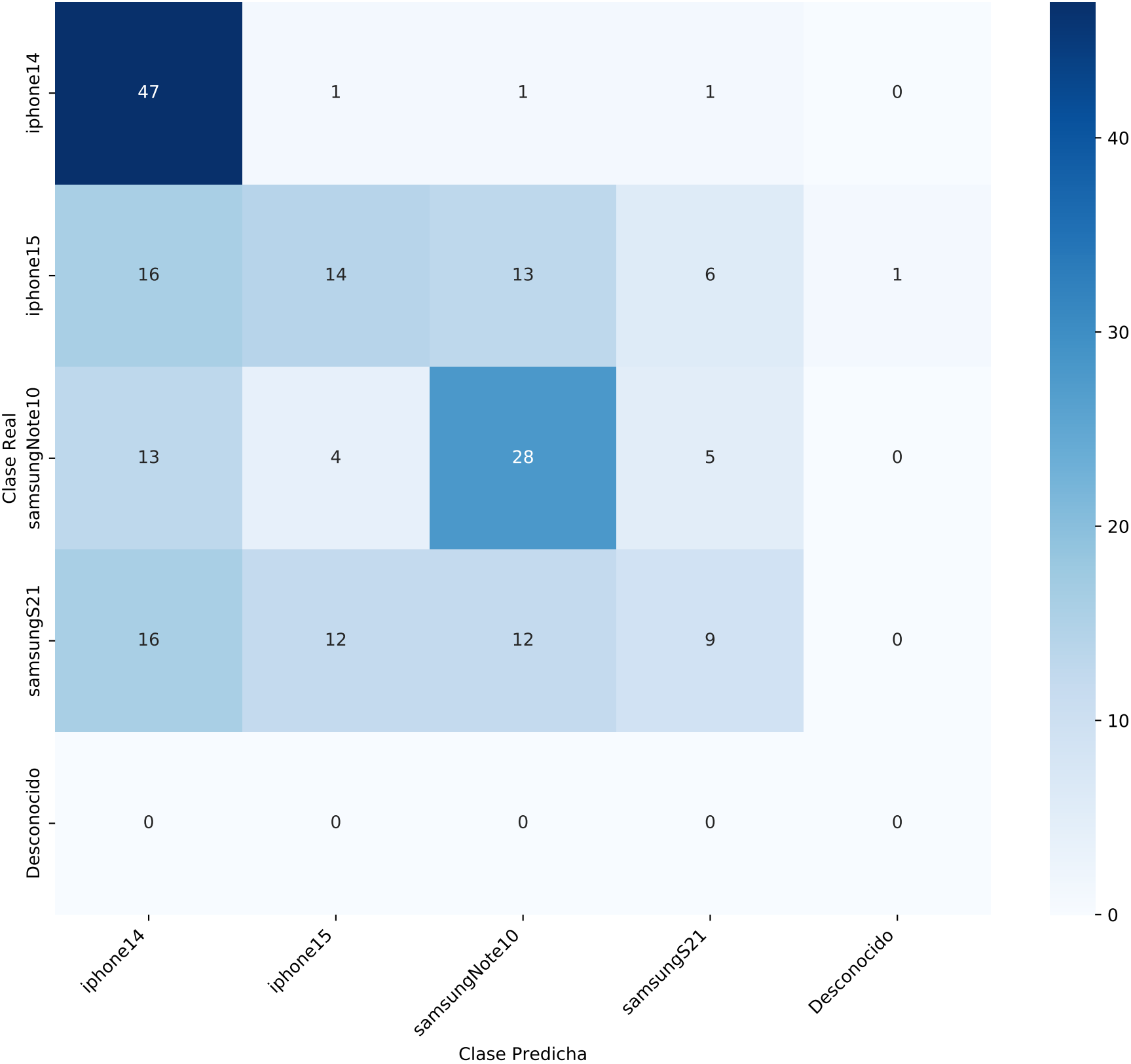
Matriz de Confusión - PRNU_FILTRO LINEAL
